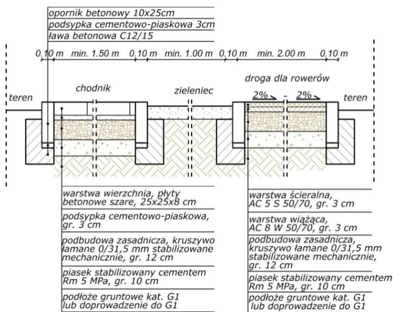
Rys. 10. Przekrój poprzeczny konstrukcji z zastosowaniem separatora w formie pasa zieleni między chodnikiem a drogą dla rowerów
