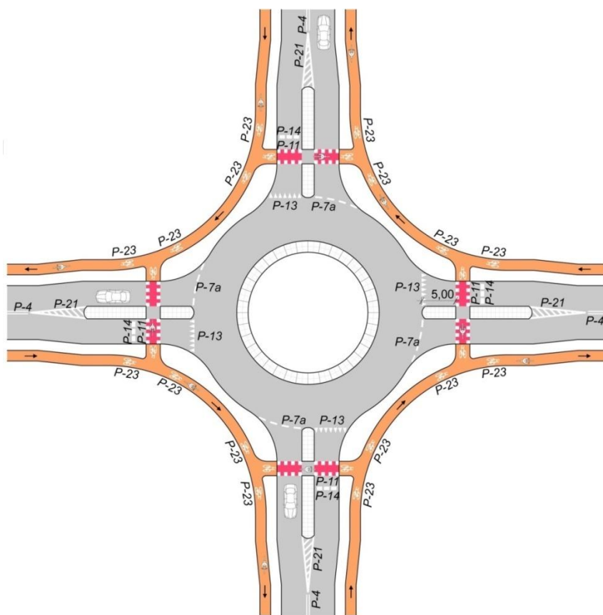
Rys. 31. Rondo z jednokierunkowymi drogami dla rowerów wokół ronda [3].
