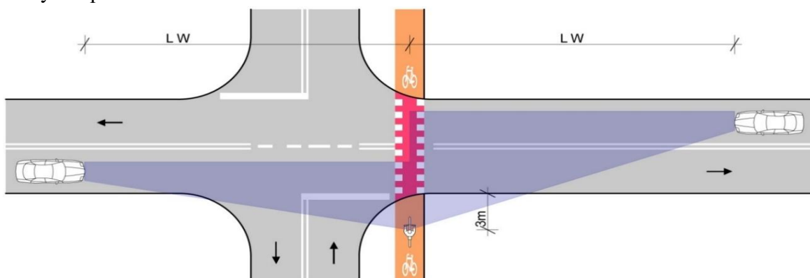
Rys. 12. Wymagana widoczność z odległości 3 metrów od krawędzi jezdni [7].
