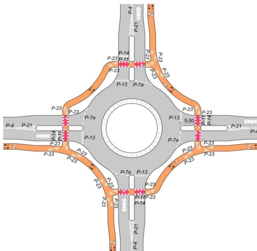
Rys. 32. Rondo z dwukierunkowymi drogami dla rowerów – dwukierunkowy ruch rowerów wokół ronda [3].
