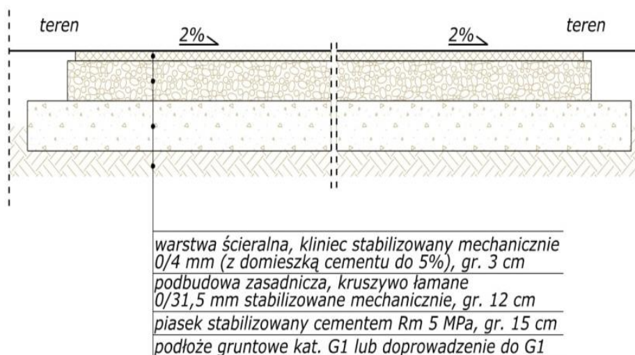
Rys. 69. Przekrój poprzeczny konstrukcji drogi dla rowerów (nawierzchnia gruntowa - wzmocniona).
