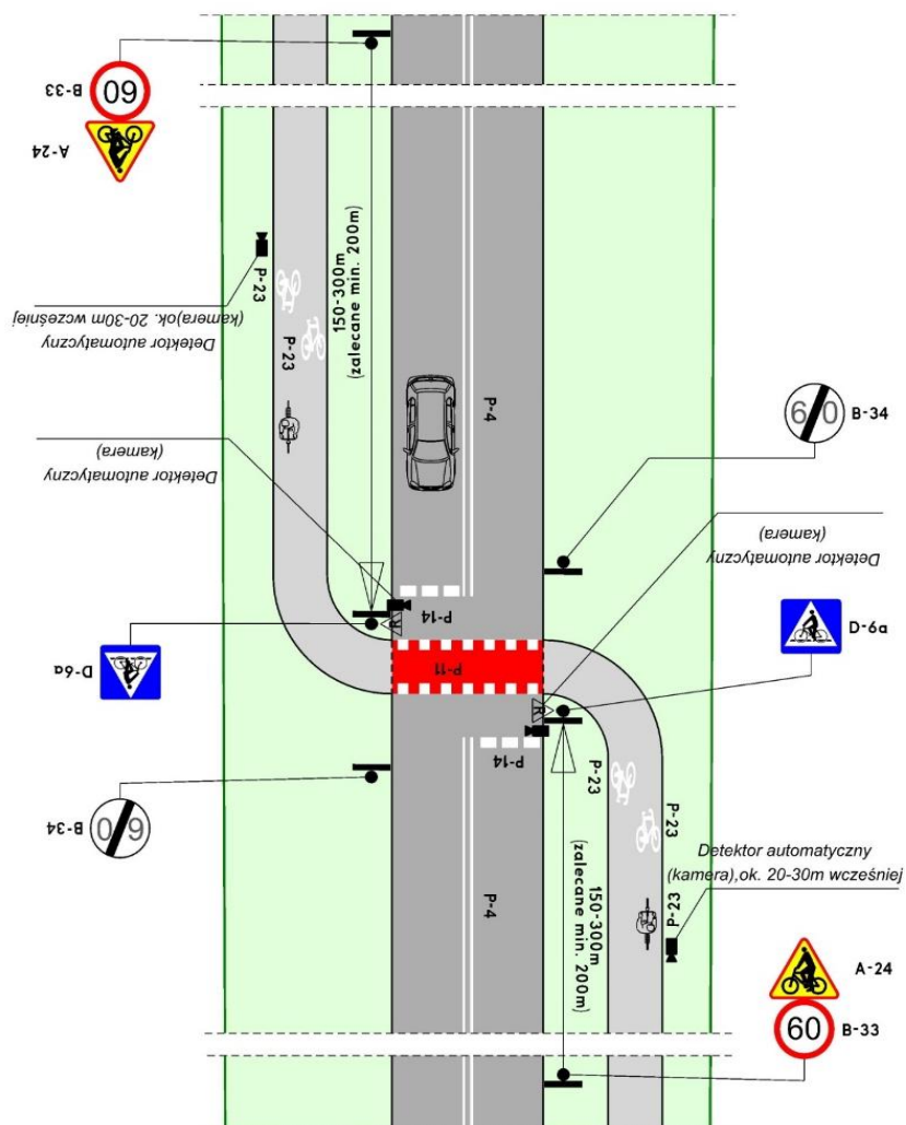
Rys. 90. Zastosowanie detektora ruchu rowerowego – detektor automatyczny (kamera).
