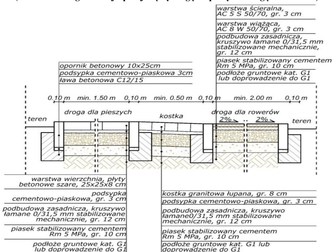
Rys. 72. Przekrój poprzeczny konstrukcji z zastosowaniem separatora w formie kostki granitowej łupanej między drogą dla pieszych a drogą dla rowerów.
