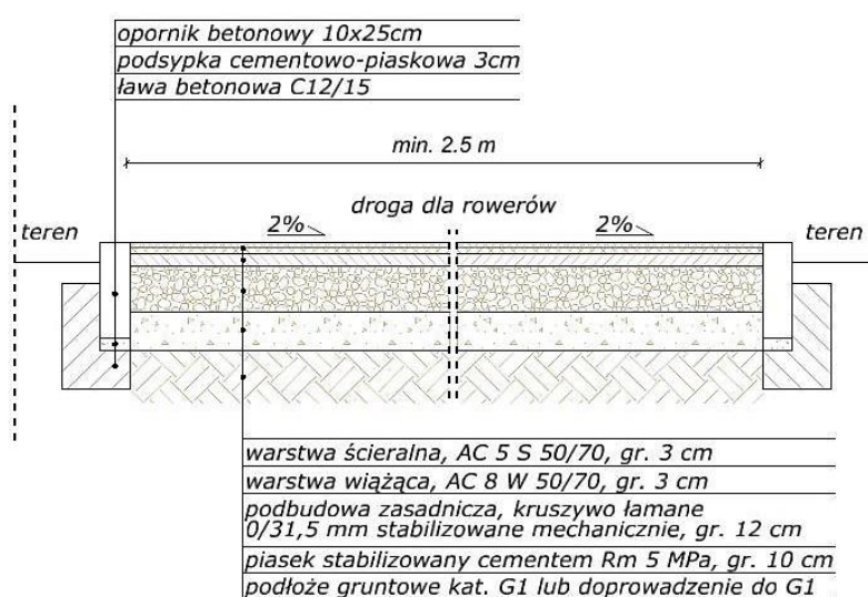
Rys. 5. Przekrój poprzeczny konstrukcji drogi dla rowerów i pieszych (nawierzchnia asfaltowa).
