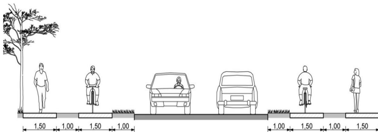
Rys. 7. Przykład separacji jednokierunkowych dróg dla rowerów w przekroju ulicy [2].
