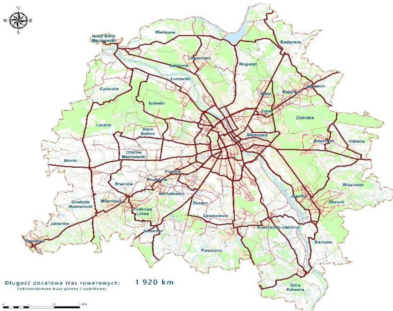
Rys. 2. Planowana sieć tras rowerowych o charakterze komunikacyjnym dla Warszawskiego Obszaru Funkcjonalnego.
