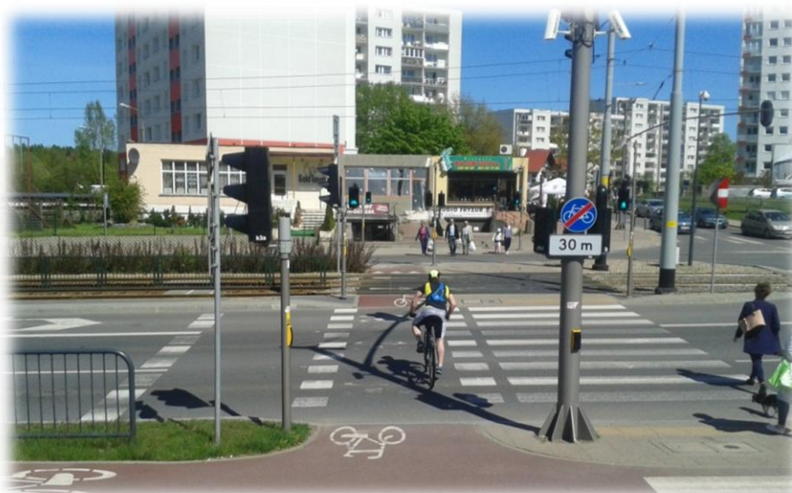
Foto 75. Zamontowane na maszcie dwie kamery, z których obraz jest analizowany w systemie sterującym sygnalizacją. Jedna kamera dostosowana do ruchu rowerowego, a druga do ruchu pieszego.
