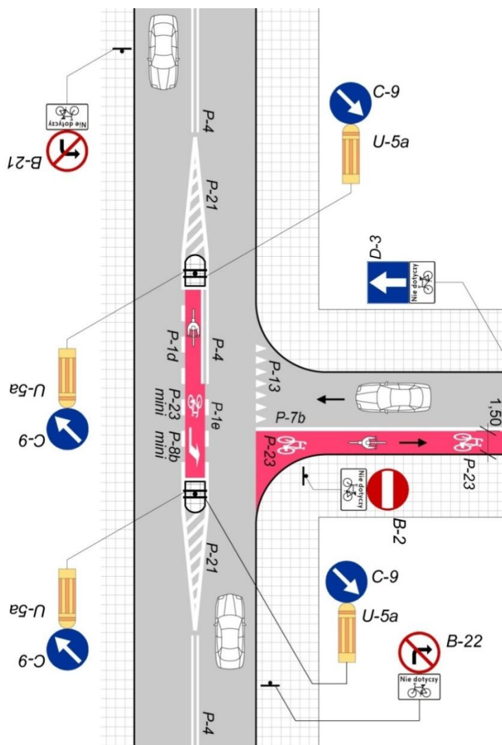
Rys. 34. Azyl dla rowerzystów na skrzyżowaniu do skrętu w lewo na kontrapas.
