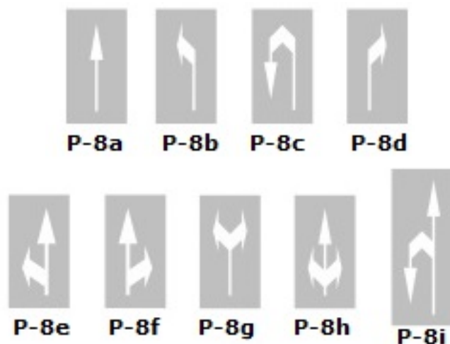
Rys. 86. Wzory znaków poziomych – strzałki, stosowane na śluzach dla rowerów.
