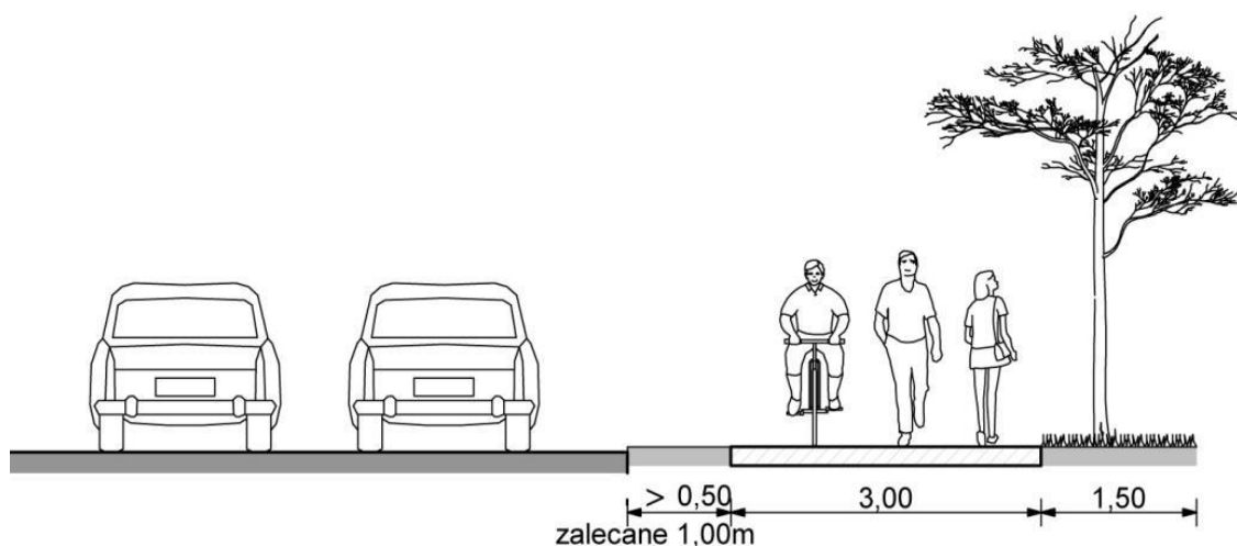
Rys. 3. Przykład usytuowania drogi dla rowerów i pieszych odseparowanej od jezdni [1].
