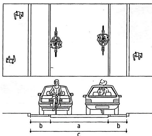
Rys. 103. Ulica rowerowa z ruchem rowerowym na pasie w środku jezdni (tzw. sugerowanym pasie ruchu dla rowerów). Jezdnia o szerokości 4,5-5,0 m, pasy zewnętrzne o szerokości 0,75 m, wydzielające dwukierunkowy pas ruchu dla rowerów o szerokości 3,0-3,5 m. Zaleca się, aby parkowanie było dopuszczalne tylko poza jezdnią.
