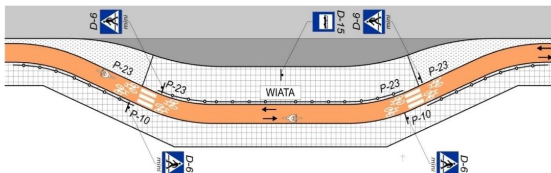
Rys. 40. Droga dla rowerów przy zatoce autobusowej [4].
