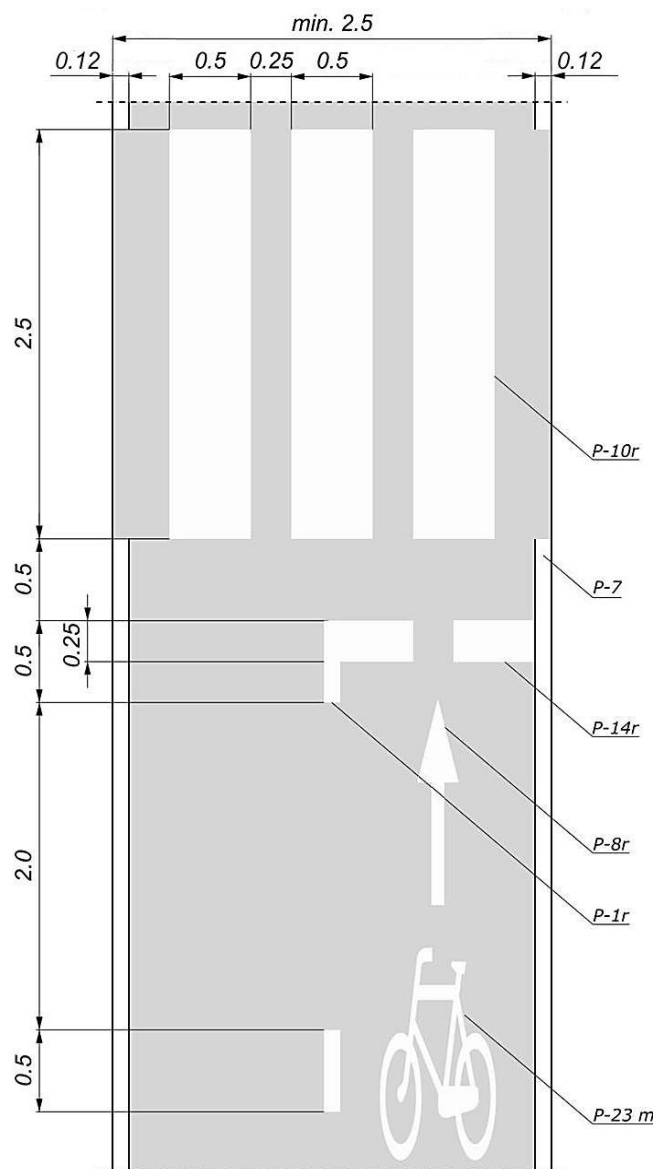
Rys. 99. Schemat oznakowania poziomego dwukierunkowej drogi dla rowerów z przejściem dla pieszych.
