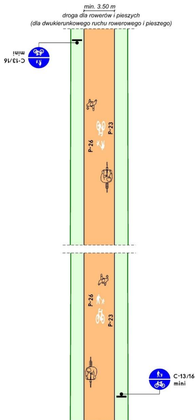
Rys. 6. Droga dla rowerów i pieszych (dla dwukierunkowego ruchu rowerowego i pieszego). Zastosowanie znaków: pionowych C-13/16 mini oraz poziomych P-23 i P-26.
