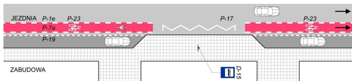
Rys. 43. Pas ruchu dla rowerów przy pasie do parkowania z przerwą na przystanek autobusowy [4].
