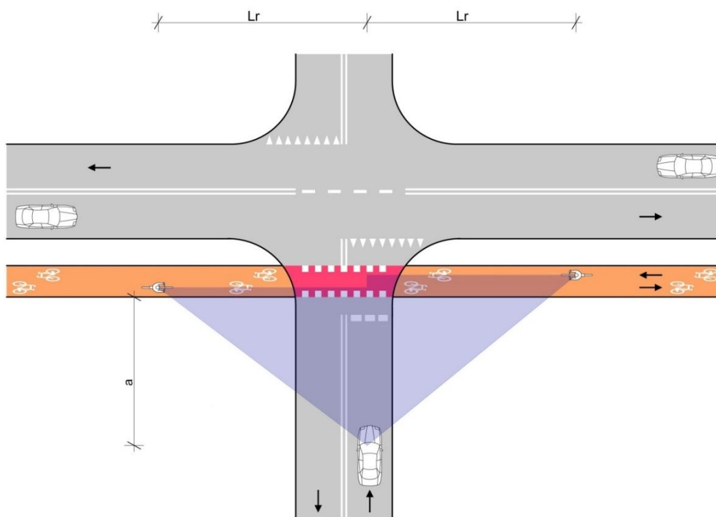
Rys. 13. Przykład zachowania widoczności na skrzyżowaniu z przejazdem dla rowerzystów [7].
