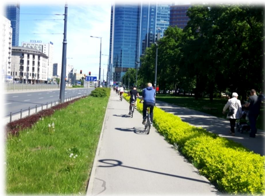
Foto 12. Zielen niska (liściasta) w pasie między drogą dla rowerów a chodnikiem. Separacja zastosowana na głównej drodze dla rowerów o funkcji komunikacyjnej. Trasa łączy przedmieścia, dzielnice i centrum miasta.
