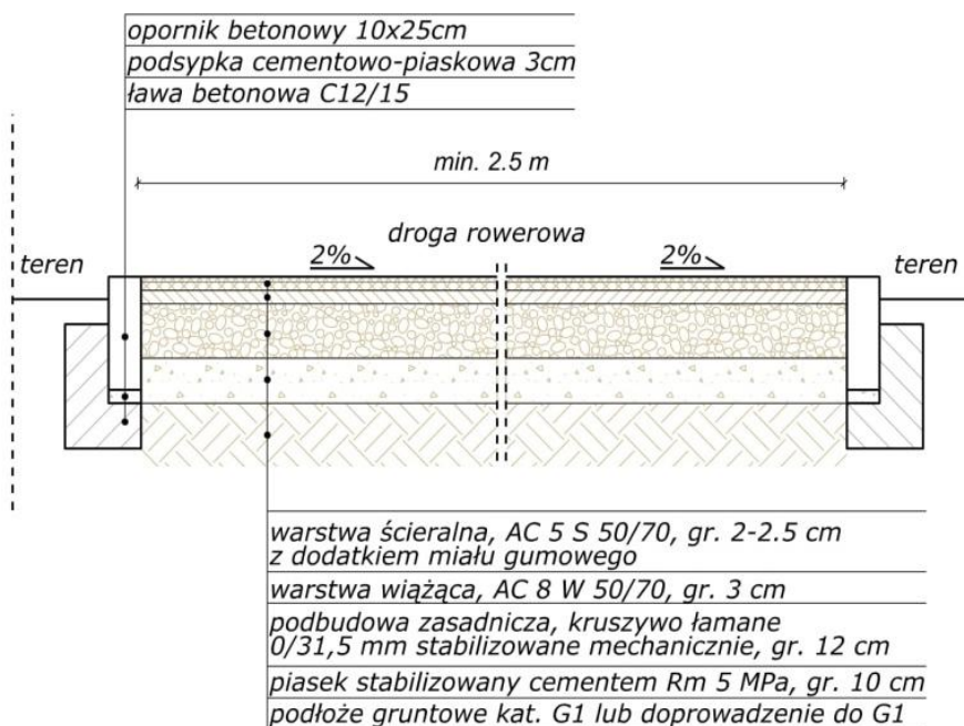
Rys. 67. Przekrój poprzeczny konstrukcji drogi dla rowerów (nawierzchnia asfaltowa z dodatkiem mialu gumowego).
