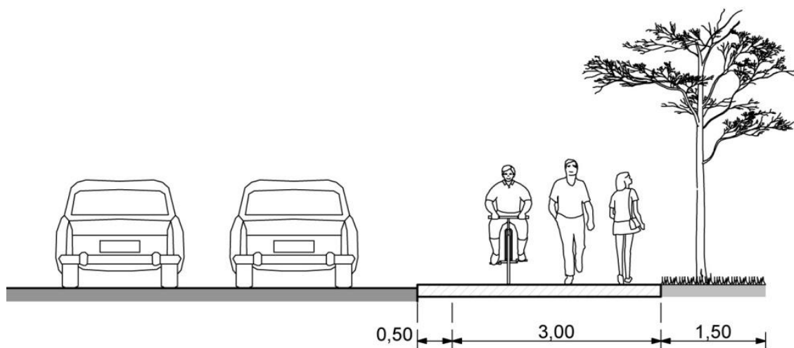
Rys. 4. Przykład usytuowania drogi dla rowerów i pieszych przylegającej do jezdni [1].
