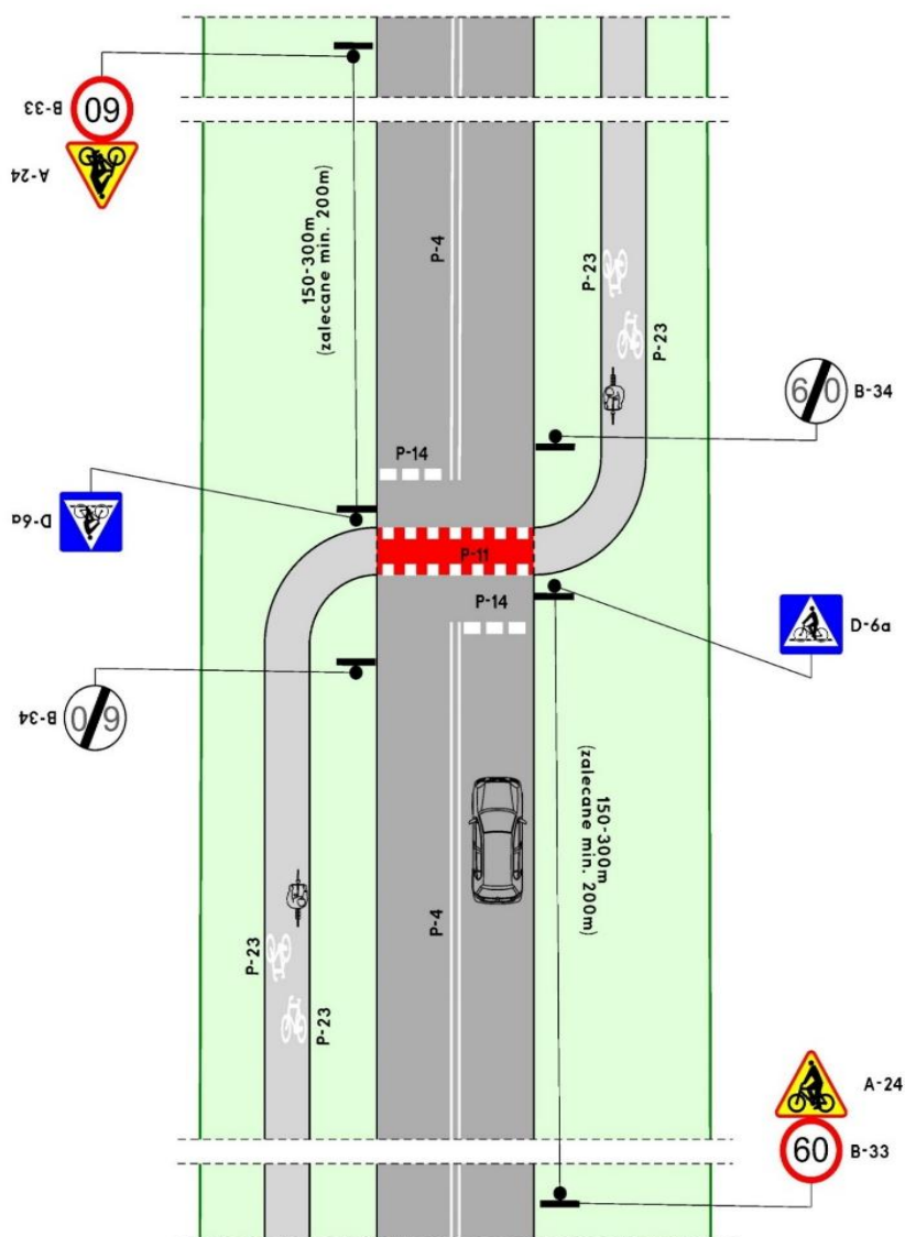
Rys. 59. Schemat przejazdu dla rowerzystów poza obszarem zabudowanym.
