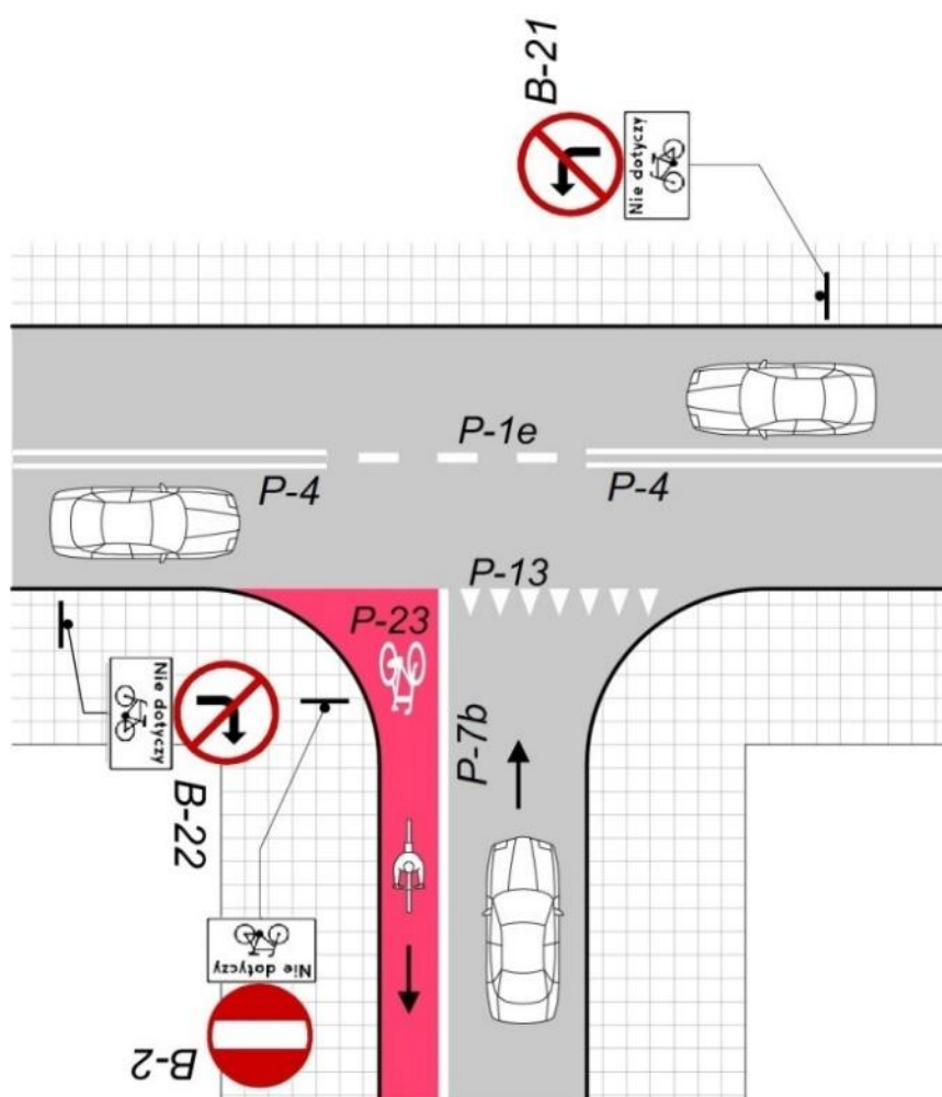
Rys. 26. Początek kontrapasu na skrzyżowaniu. Zastosowanie oznakowania poziomego P-23, P-13 oraz oznakowania pionowego B-22, B-2 i linii P-7b.
