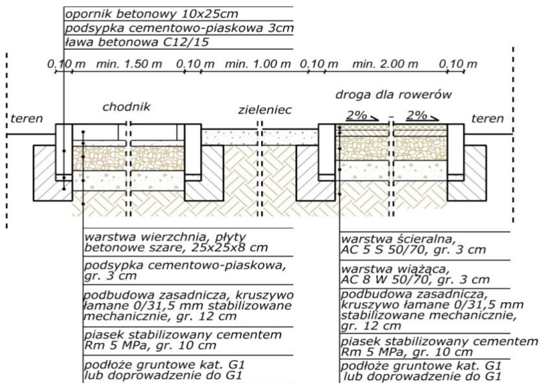
Rys. 71. Przekrój poprzeczny konstrukcji z zastosowaniem separatora w formie pasa zieleni między chodnikiem a drogą dla rowerów
