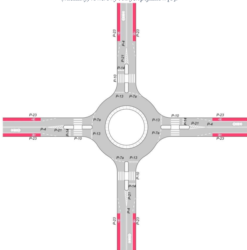
Rys. 30. Małe rondo – pasy ruchu dla rowerów przed i za rondem, na rondzie ruch na zasadach ogólnych (mieszany) rowerowy i innych pojazdów [3].
