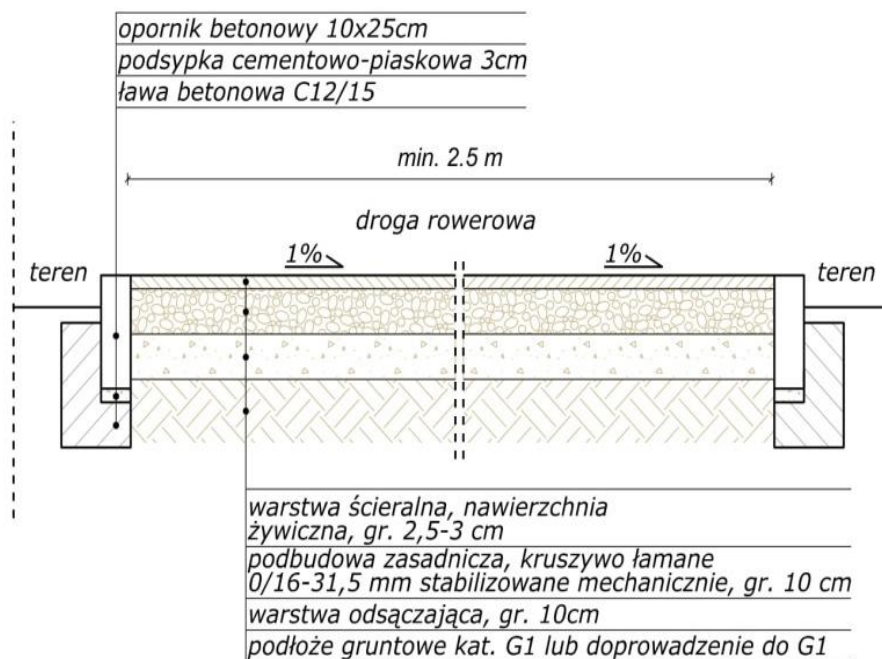
Rys. 68. Przekrój poprzeczny konstrukcji drogi dla rowerów (nawierzchnia wodoprzepuszczalna żywiczna).
