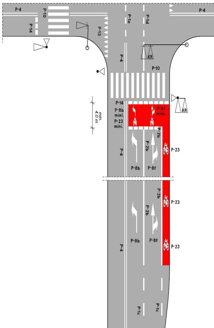
Rys. 23. Śluzka dla rowerów – dwupasowy wlot na skrzyżowaniu z segregacją kierunków ruchu. Śluzka umożliwia jazdę ze skrzyżowania w lewo, na wprost i w prawo.
