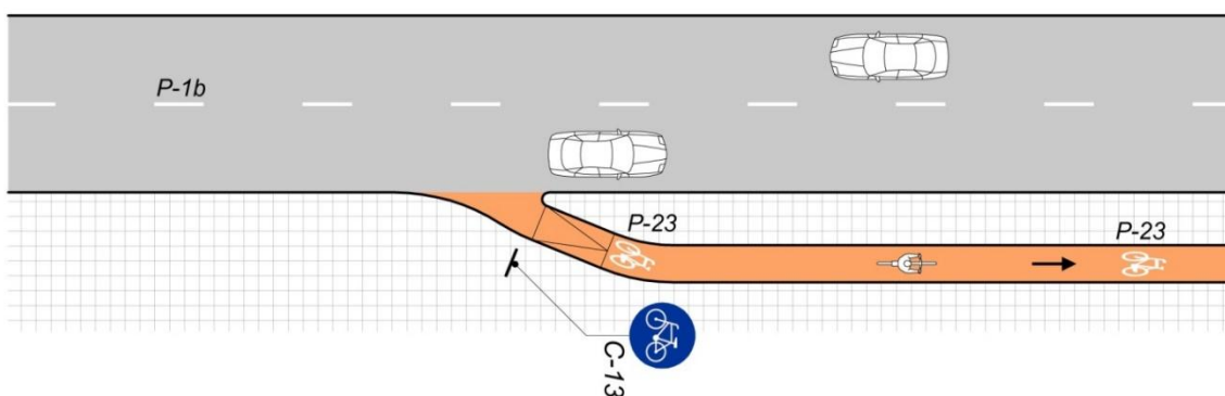
Rys. 39. Wjazd z jezdni (ruch mieszany na zasadach ogólnych) na jednokierunkową drogę dla rowerów
