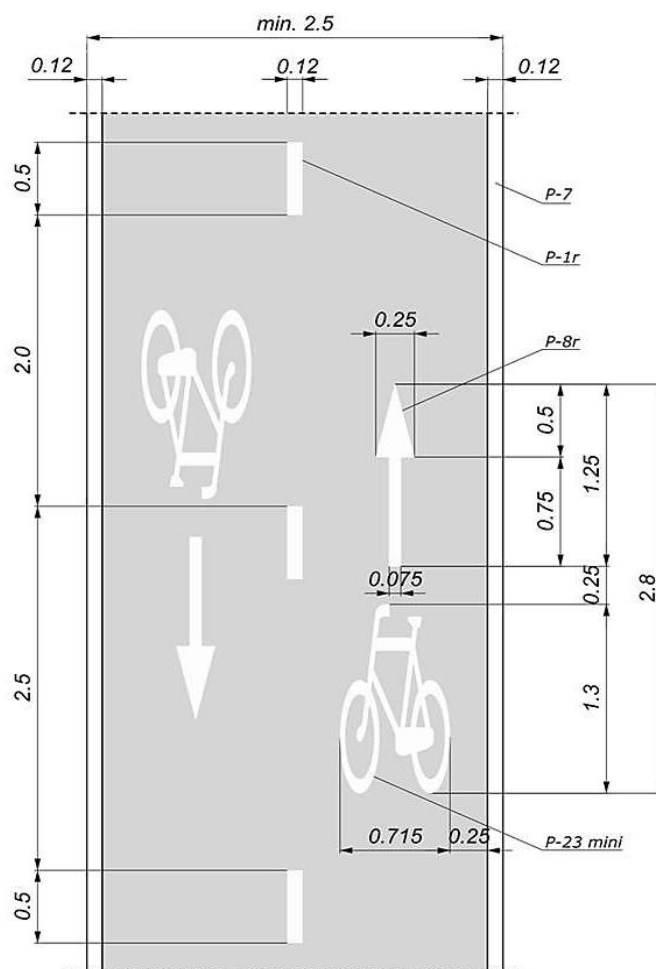
Rys. 98. Schemat oznakowania poziomego dwukierunkowej drogi dla rowerów.
