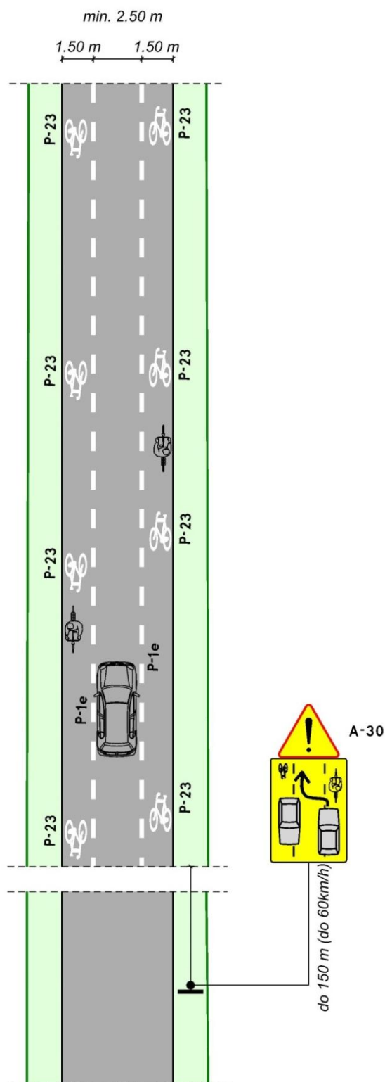
Rys. 101. Schemat przekroju „2-1” dla rowerów na drodze (ruch na zasadach ogólnych) o dopuszczalnej prędkości nie większej niż 50 km/h (zalecana 30 km/h).
