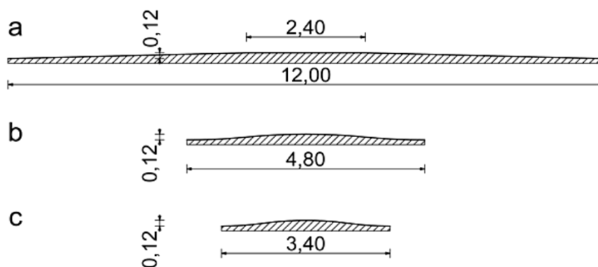
Rys. 17. Przekroje podłużne progów zwalniających sprzyjających ruchowi rowerowemu.
