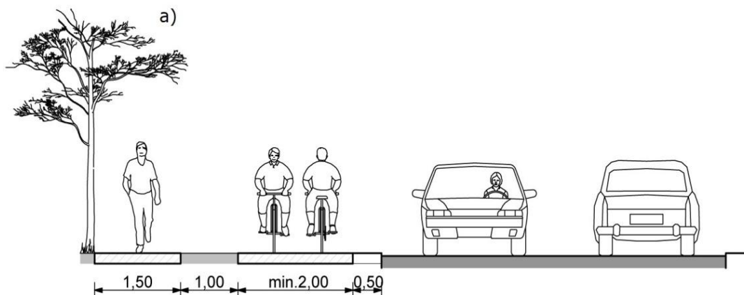
Rys. 8. Przykład separacji (trawnik) wydzielonych dwukierunkowych dróg dla rowerów w przekroju ulicy [2].
