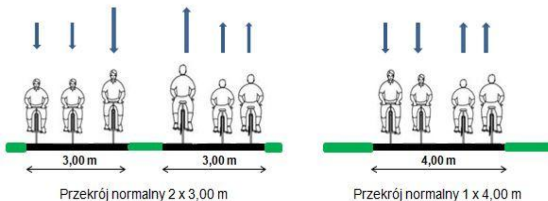
Rys. 100. Schemat rowerostrad zgodnie ze standardami krajowymi (2019) i holenderskimi (2016).
