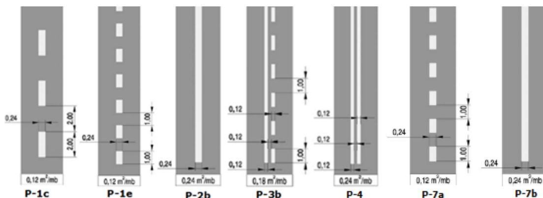
Rys. 85. Wzory znaków poziomych – linie rozdzielające pasy.
