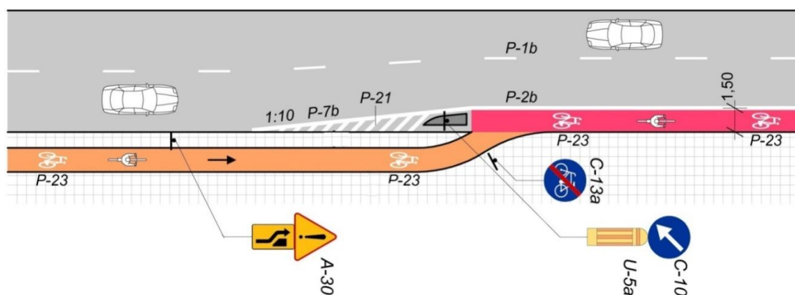
Rys. 35. Zjazd z jednokierunkowej drogi dla rowerów na jednokierunkowy pas ruchu dla rowerów:
