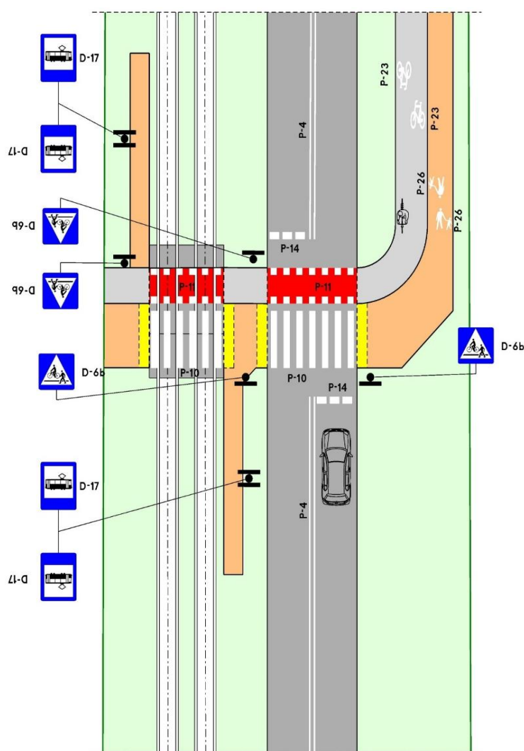
Rys. 64. Schemat przejazdu rowerowego przez torowisko tramwajowe.
