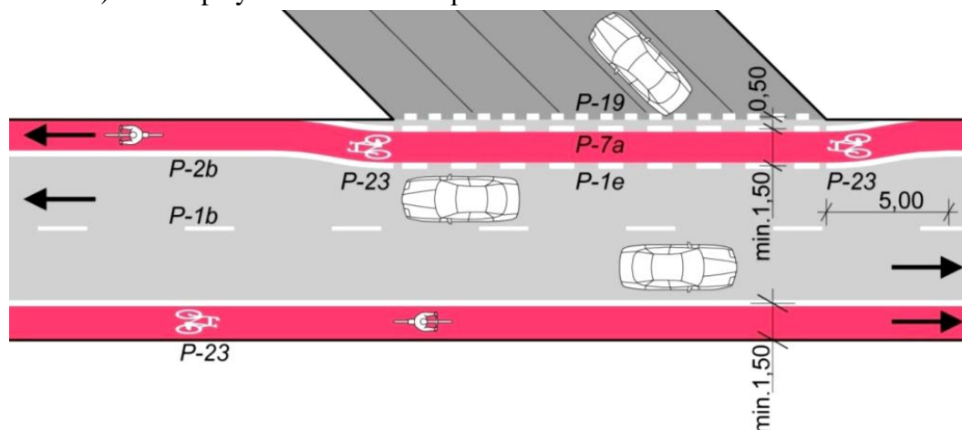
Rys. 20. Pasy ruchu dla rowerów po obu stronach na jezdni dwukierunkowej [4].
