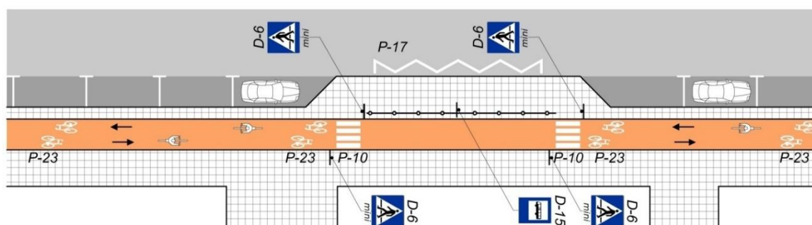
Rys. 41. Droga dla rowerów przy pasie do parkowania i przystanku autobusowym [4].
