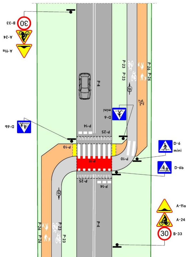
Rys. 61. Schemat przejazdu dla rowerzystów na płytowym progu zwalniającym połączony z przejściem dla pieszych.
