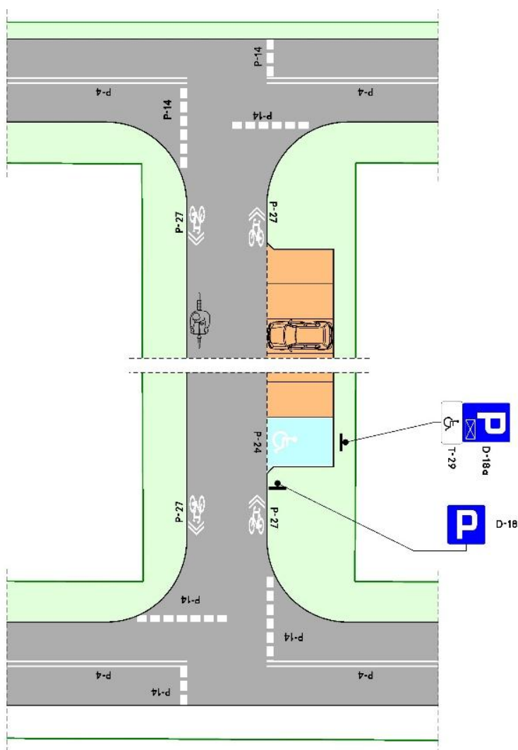
Rys. 14. Ruch rowerowy na zasadach ogólnych z zastosowaniem znaku P-27.
