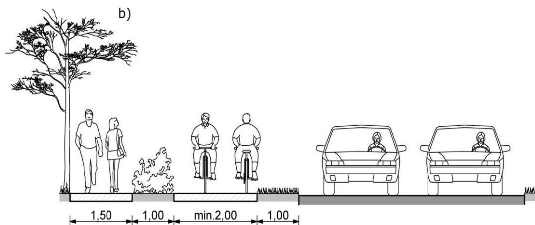
Rys. 9. Przykład separacji (niski żywopłot) wydzielonej dwukierunkowej drogi dla rowerów w przekroju ulicy [2].
