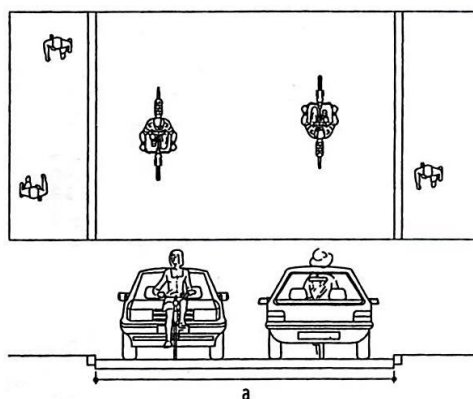
Rys. 102. Ulica rowerowa z przekrojem dla ruchu mieszanego. Jezdnia o szerokości min. 4,5 m.
