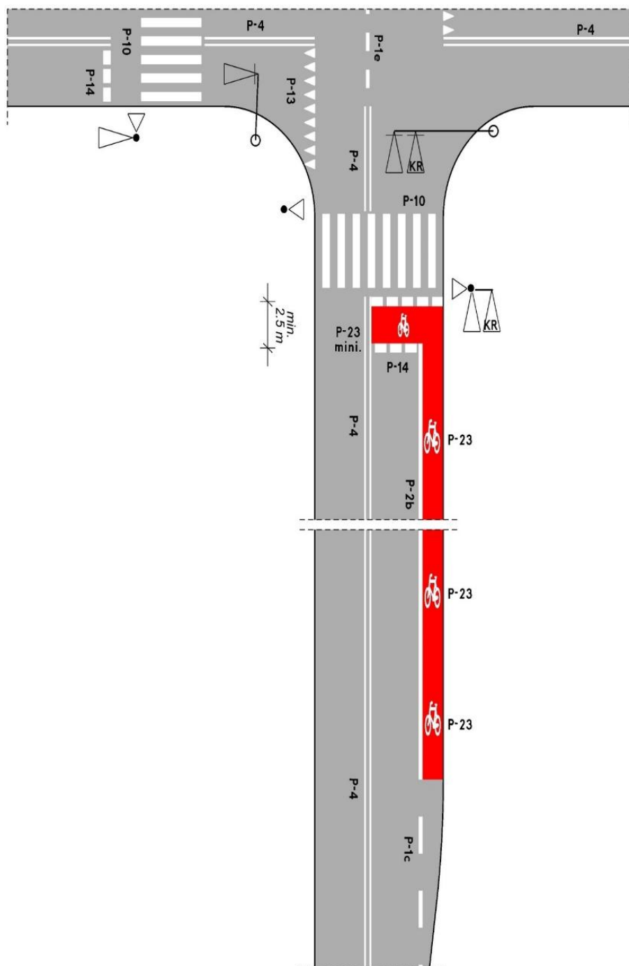
Rys. 24. Śluzka dla rowerów – jednopasowy wlot na skrzyżowaniu.
