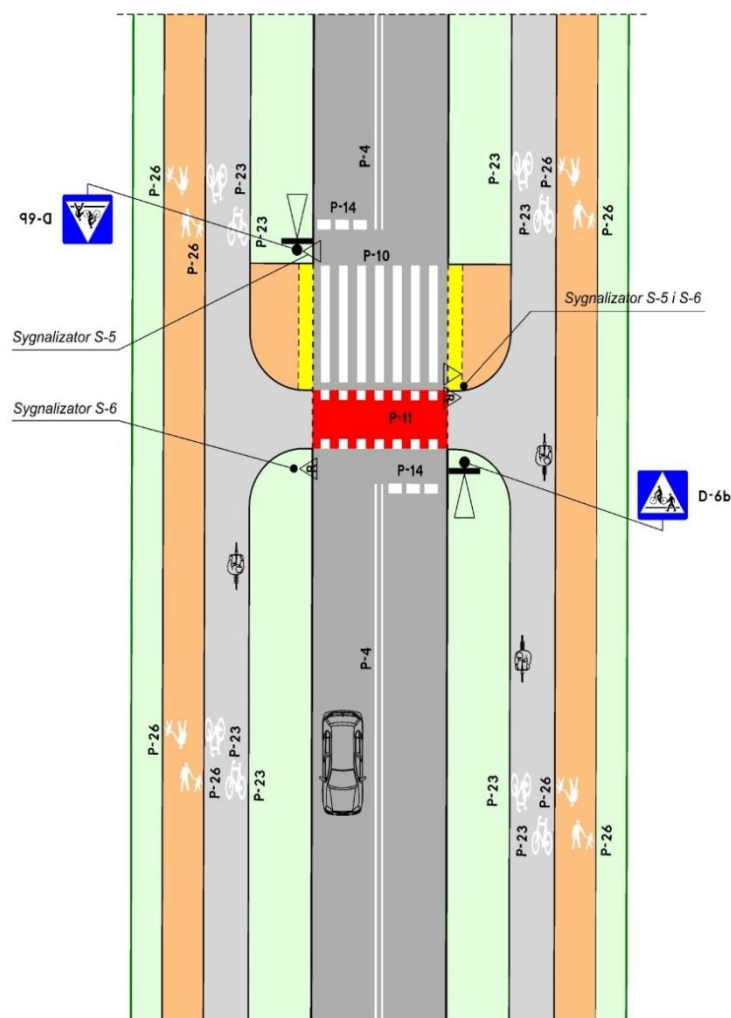
Rys. 92. Umieszczenie sygnalizatorów na przejazdach dla rowerzystów
