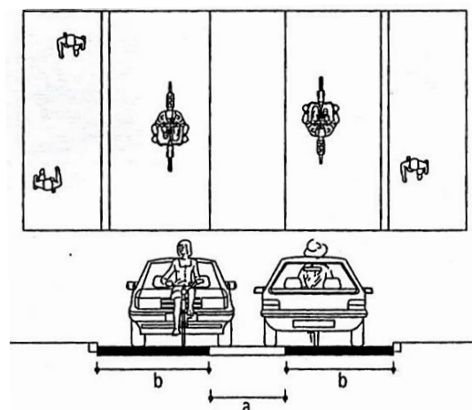
Rys. 104. Ulica rowerowa z pasem dzielącym jezdnię i ruchem rowerowym na zewnątrz jezdni. Jezdnia o szerokości min. 5,5 m, z pasami ruchu dla rowerów po zewnętrznych stronach jezdni o szerokości 2,25 m oraz przejezdnym pasem środkowym o szerokości min. 1,0 m.
