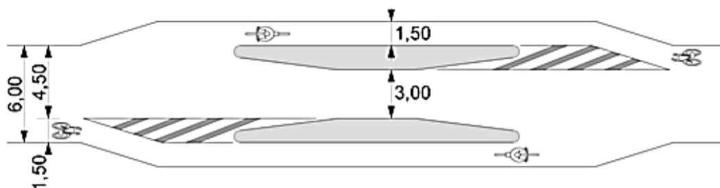
Rys. 15. Organizacja ruchu rowerowego poprzez zastosowanie pasów ruchu dla rowerów, omijających próg zwalniający na ulicy w strefie ruchu uspokojonego [6].
