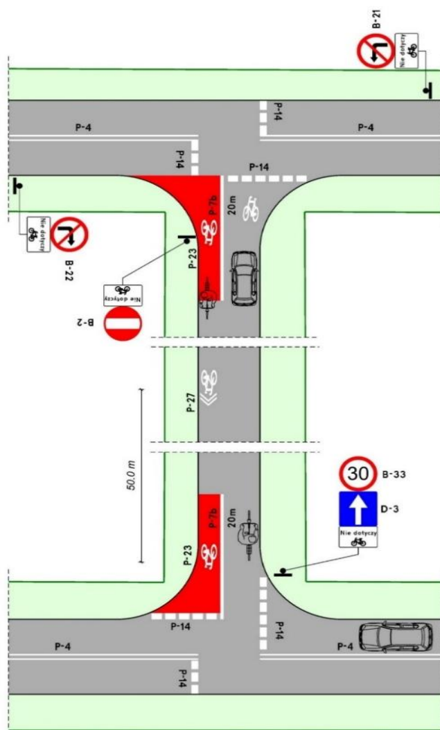
Rys. 19. Zastosowanie kontraruchu przy dopuszczalnej prędkości 30 km/h na drogach klasy (L) i dojazdowych (D).
