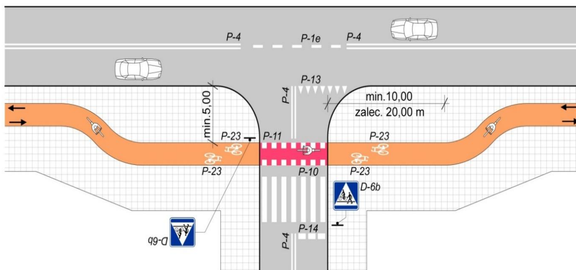
Rys. 21. Droga dla rowerów z odgięciem toru jazdy (20 m) od skrzyżowania [5].
