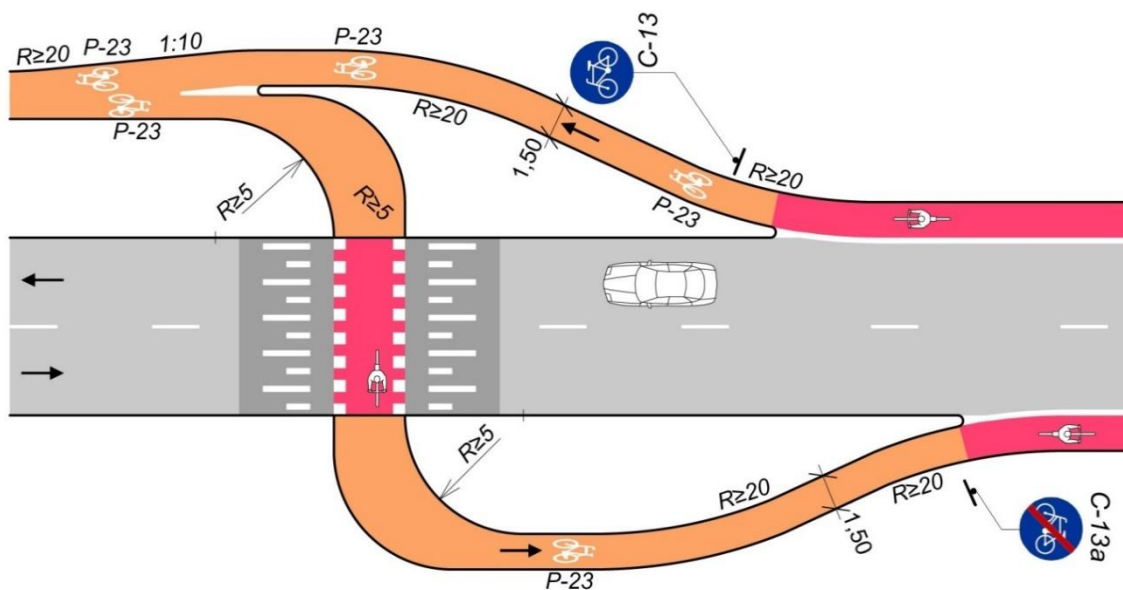
Rys. 37. Zjazd z dwukierunkowej drogi dla rowerów na jednokierunkowy pas ruchu dla rowerów oraz zjazd z pasa ruchu dla rowerów na drogę dla rowerów
