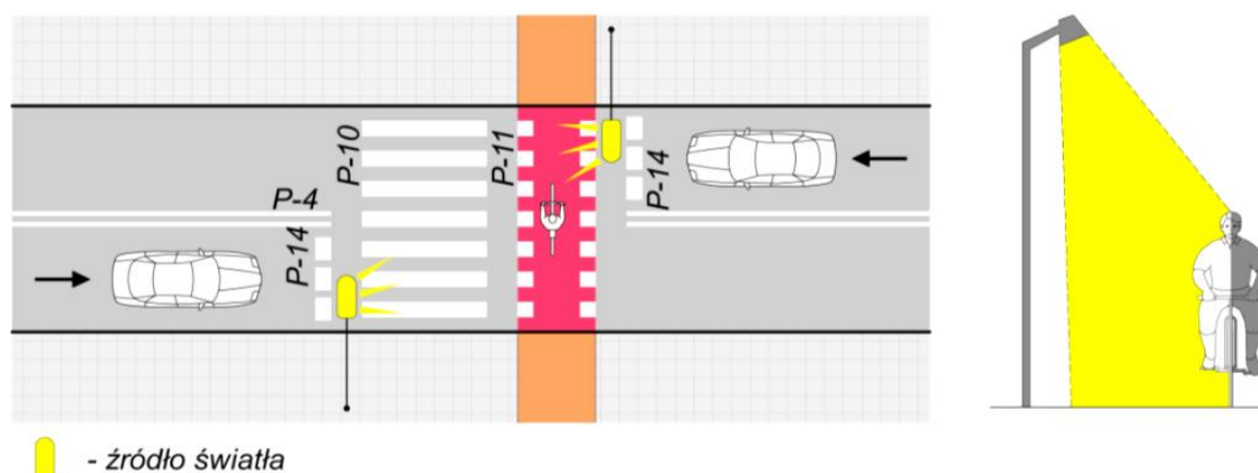
Rys. 89. Schemat prawidłowo usytuowanego oświetlenia przejścia dla pieszych i przejazdów dla rowerzystów
