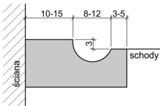
Rys. 96. Zalecany przekrój poprzeczny prowadnicy wg Wytycznych organizacji bezpiecznego ruchu rowerowego (2019) oraz holenderskich standardów C.R.O.W. (2016).
