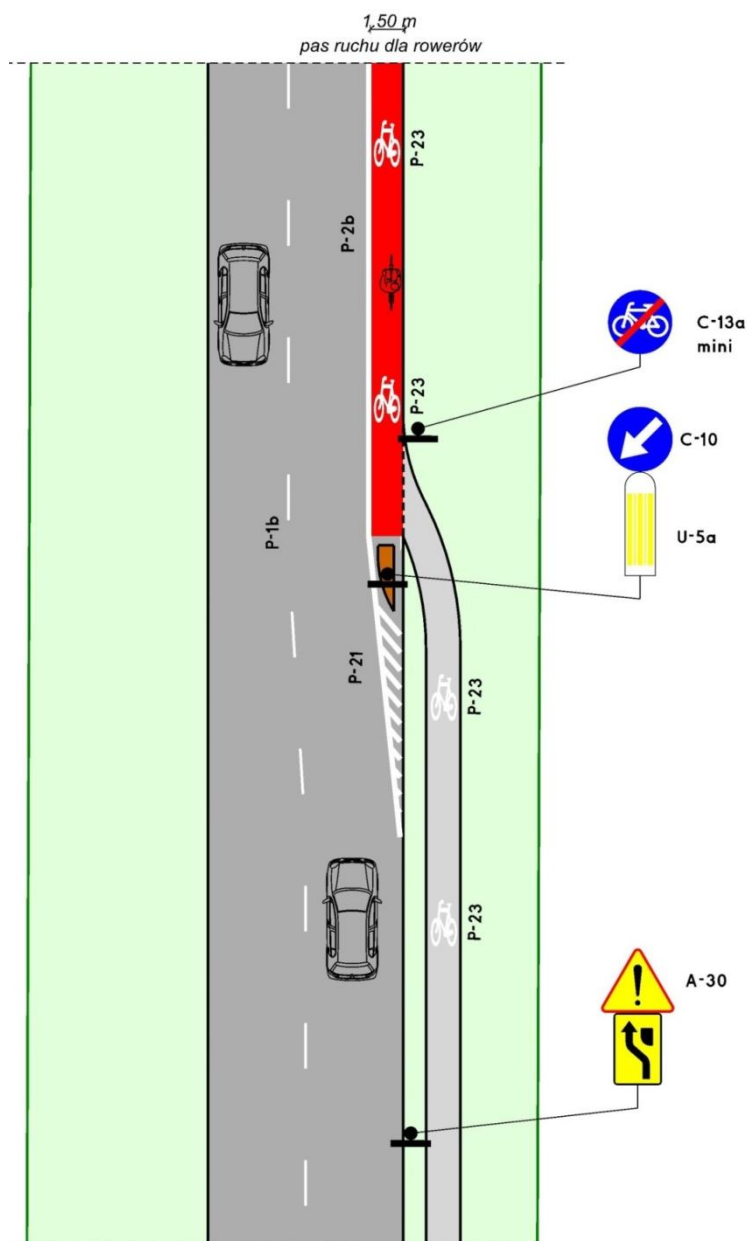
Rys. 22. Zjazd z jednokierunkowej drogi dla rowerów na jednokierunkowy pas ruchu dla rowerów zlokalizowany na jezdni [5].
