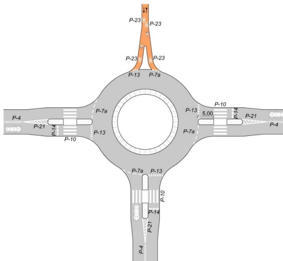
Rys. 28. Rondo małe – dwukierunkowa droga dla rowerów jako dodatkowy wlot na rondo, na rondzie ruch na zasadach ogólnych (ruch mieszany) rowerowy i innych pojazdów [3].
