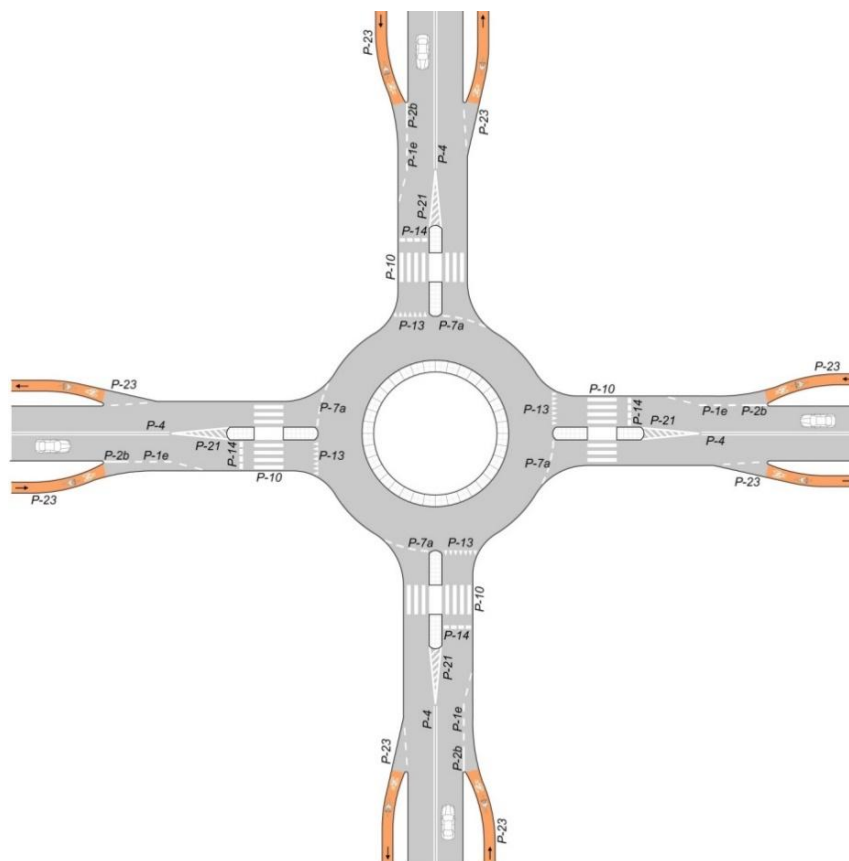
Rys. 29. Małe rondo – zasady prowadzenia drogi dla rowerów przez i za rondem, na rondzie ruch na zasadach ogólnych (mieszany) rowerowy i innych pojazdów [3].
