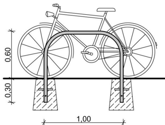
Rys. 94. Rekomendowany stojak dla rowerów wg Wytoczny organizacji bezpiecznego ruchu rowerowego (2019) oraz Standardów projektowych i wykonawczych dla infrastruktury rowerowej Województwa Dolnośląskiego (2017).
