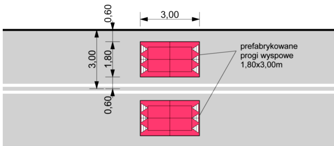
Rys. 18. Wolne przestrzennie dla swobodnego ruchu rowerów przy progach wyspowych w strefach ruchu uspokojonego [6].
