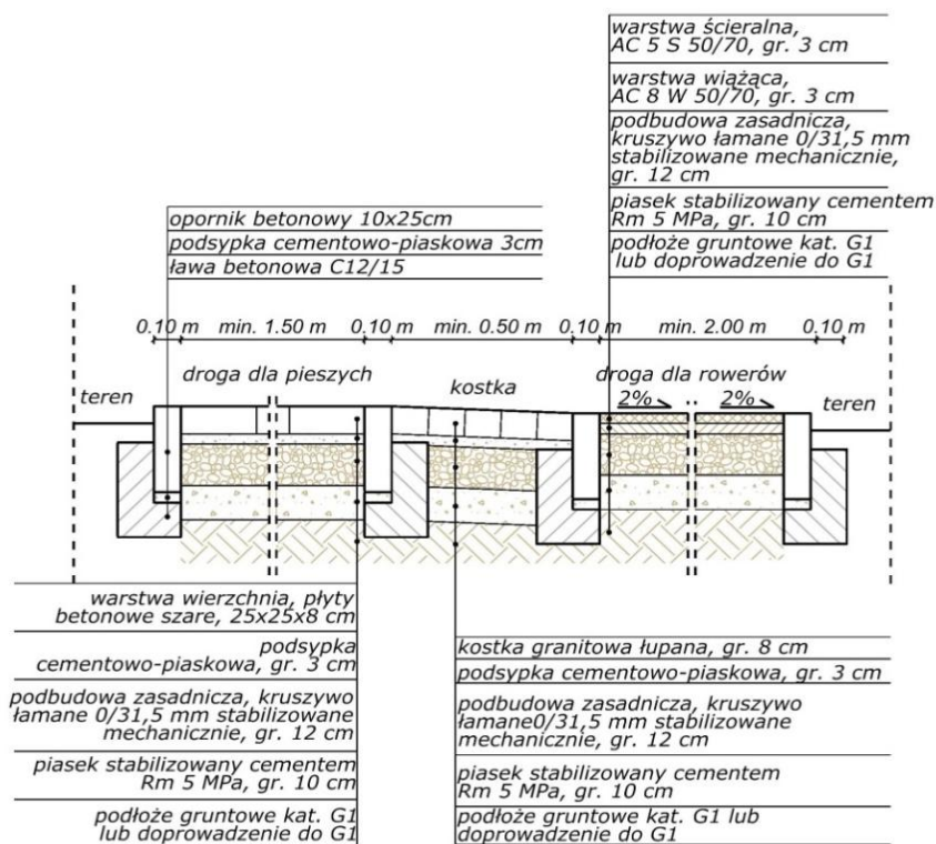
Rys. 11. Przekrój poprzeczny konstrukcji z zastosowaniem separatora w formie kostki granitowej między drogą dla pieszych a drogą dla rowerów:
