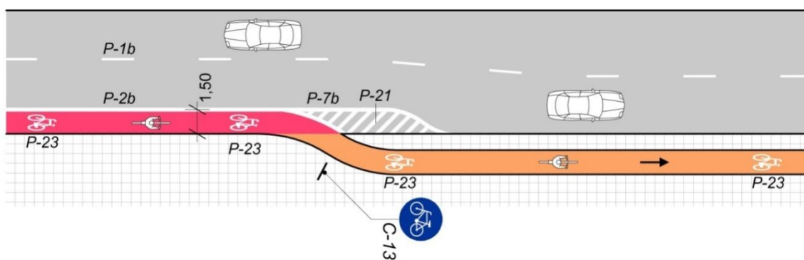
Rys. 38. Wjazd z jednokierunkowego pasa ruchu dla rowerów na jednokierunkową drogę dla rowerów
