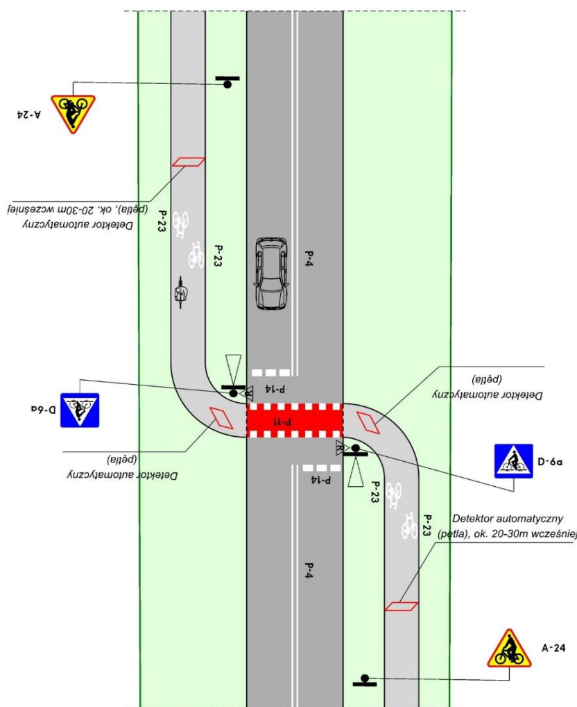
Rys. 91. Detektory ruchu rowerowego – detektor automatyczny (pętla indukcyjna).
