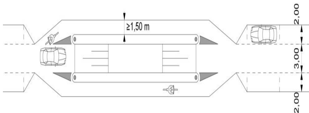
Rys. 16. Organizacja ruchu rowerowego poprzez zastosowanie pasów ruchu dla rowerów; omijających próg zwalniający na ulicy w strefie ruchu uspokojonego [6].
