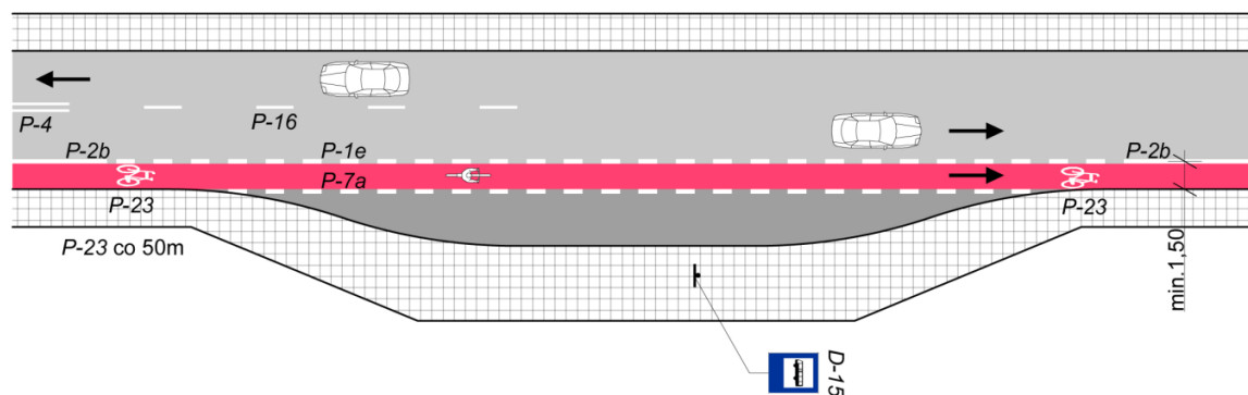
Rys. 42. Pas ruchu dla rowerów przy zatoce autobusowej [4].
