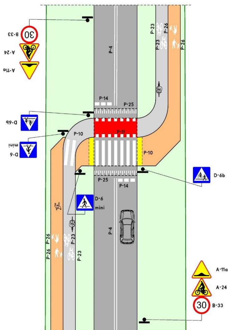
Rys. 62. Schemat przejazdu dla rowerzystów na fityowym progu zwalniającym obok przejścia dla pieszych.
