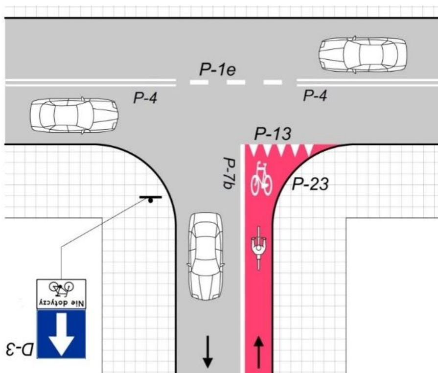
Rys. 27. Zakończenie kontrapasu, wlot na skrzyżowanie. Zastosowanie oznakowania poziomego P-23, P-7b oraz oznakowania pionowego D-3.
