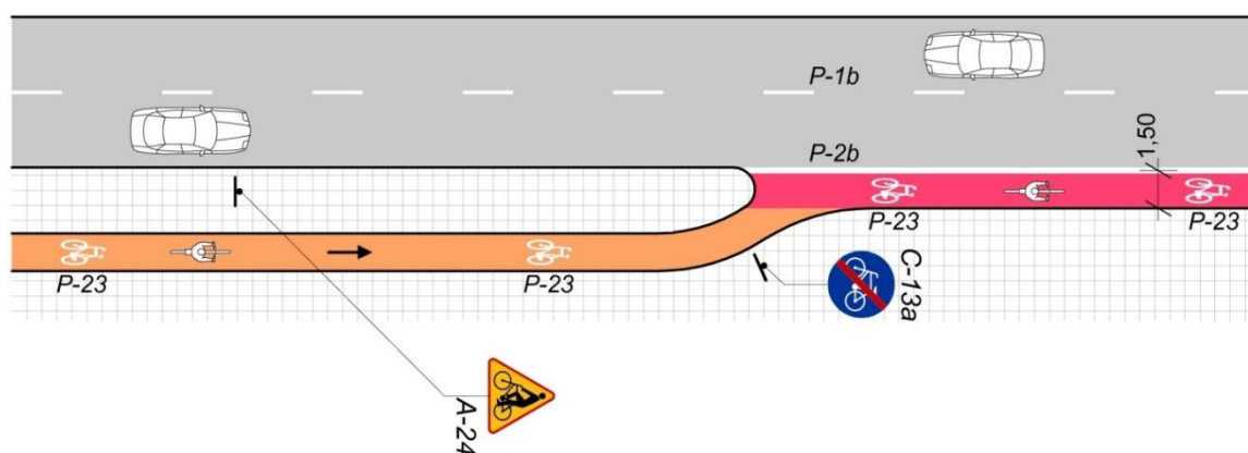
Rys. 36. Zjazd z jednokierunkowej drogi dla rowerów na jednokierunkowy pas ruchu dla rowerów; bez słupka chroniącego U-5a, ze znakiem poziomym A-24.
