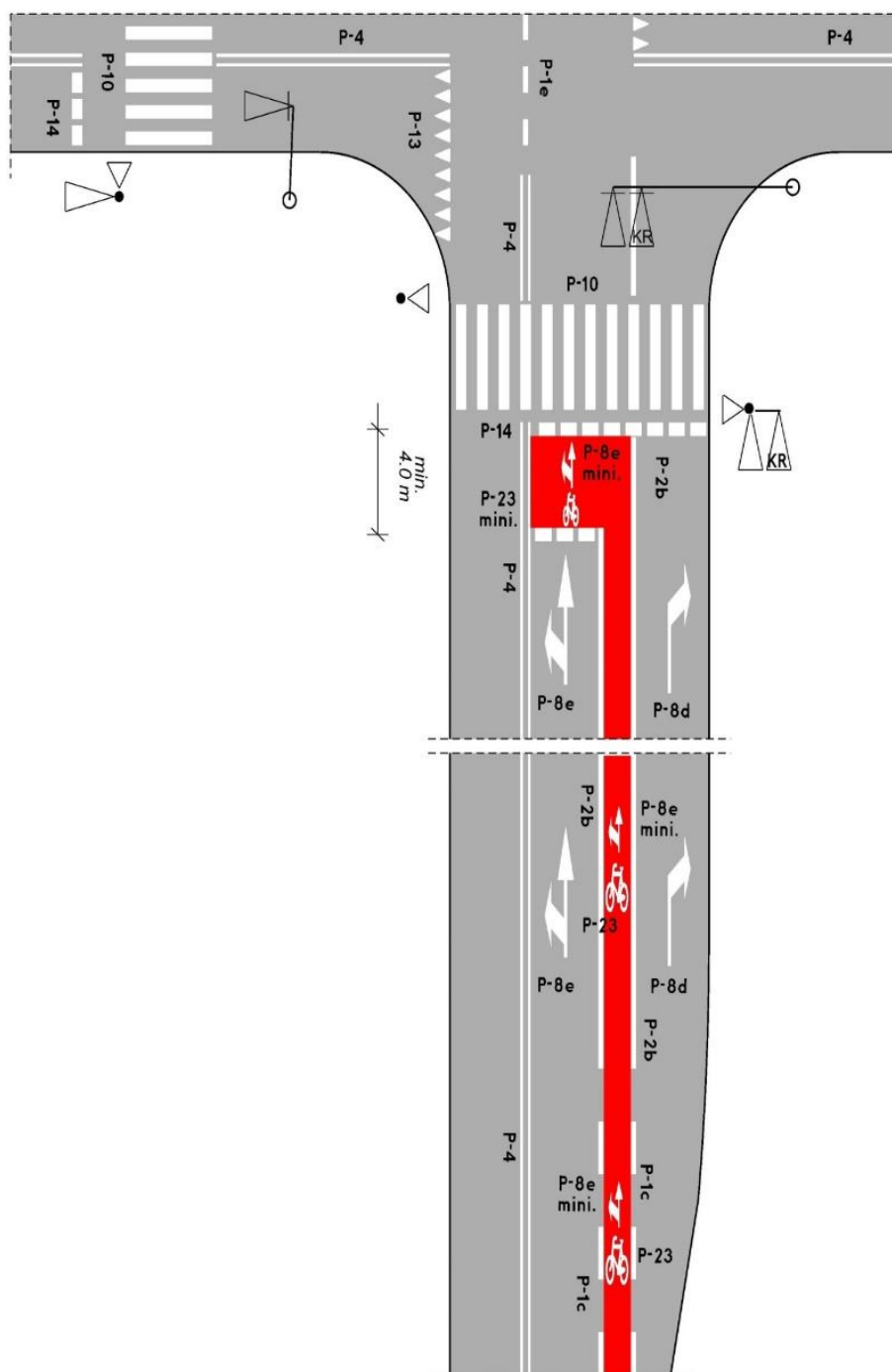
Rys. 25. Śluzka dla rowerów – wlot na skrzyżowanie z wydzielonym pasem oraz służką dla rowerów jadących na wprost i w lewo.
