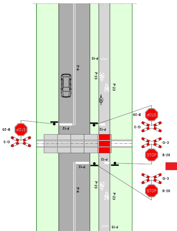
Rys. 63. Schemat przejazdu dla rowerzystów przez torowisko kolejowe w obrębie przejazdów niestrzeżonych.
