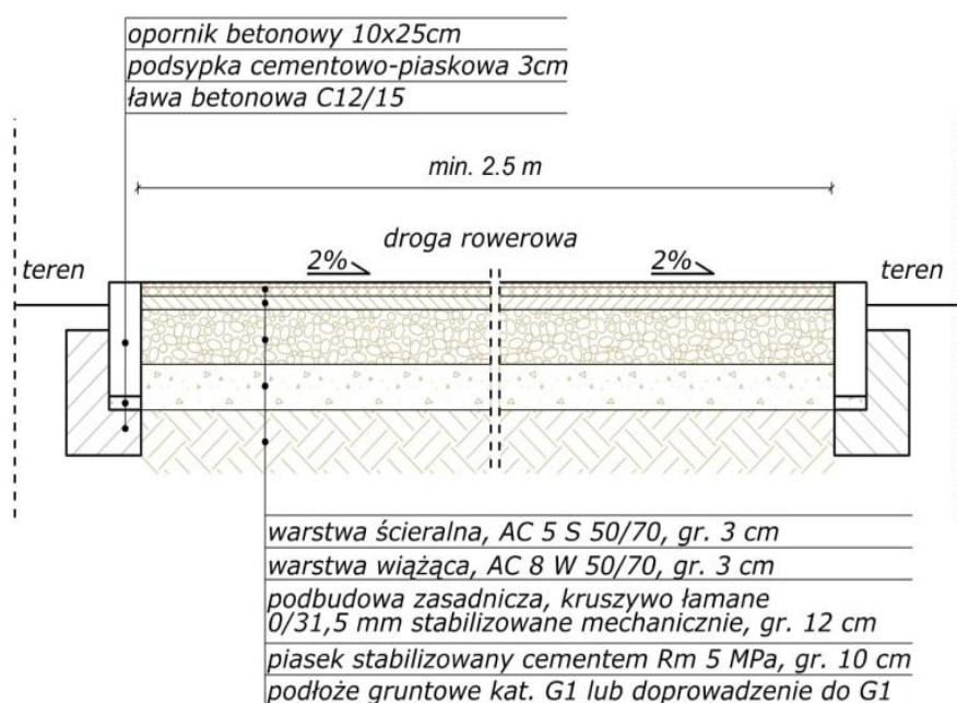
Rys. 66. Przekrój poprzeczny konstrukcji drogi dla rowerów (nawierzchnia asfaltowa).
