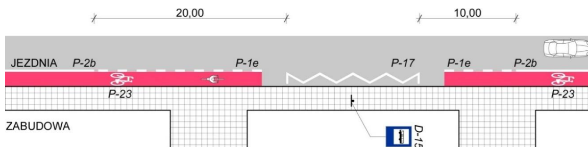
Rys. 44. Pas ruchu dla rowerów przy krawężniku z przerwą na przystanek autobusowy [4].
