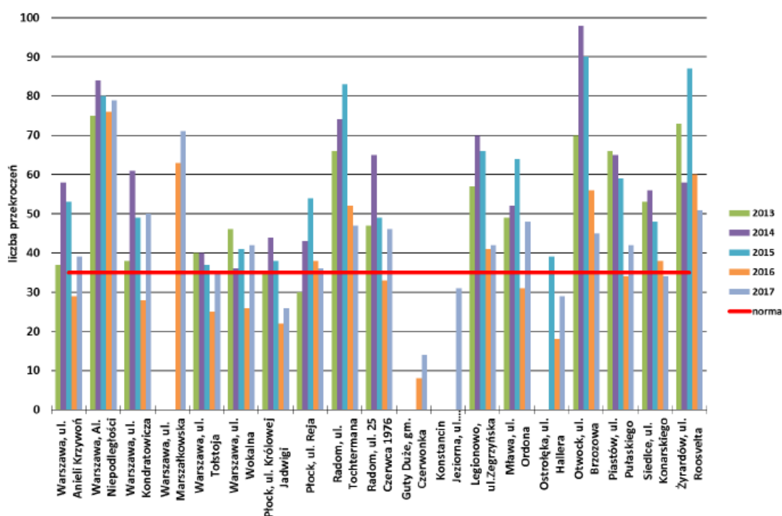
Rysunek 4.8. Częstości przekraczania dopuszczalnego poziomu stężeń 24 godzinnych pyłu zawieszonego PM10 w latach 2013 – 2017
